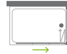
▼ TYP 5316+5317 Faltwand 3-teilig + Seitenwand 4 mm Sicherheitsglas
